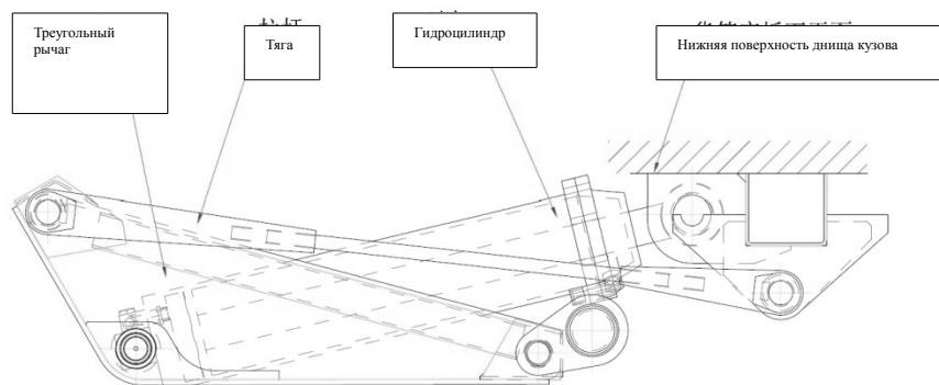
Рис.4 Подъемный механизм с конструкцией типа F
